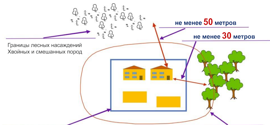
Рисунок 4. Противопожарные расстояния от зданий городских населенных пунктов до границ лесных насаждений
