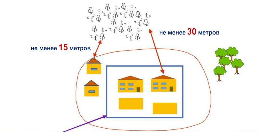
Рисунок 5. Противопожарные расстояния от зданий городских населенных пунктов в зонах индивидуальной и малоэтажной жилой застройки, от зданий и сооружений сельских населенных пунктов, а также от жилых домов на приусадебных или садовых земельных участках до границ лесных насаждений
